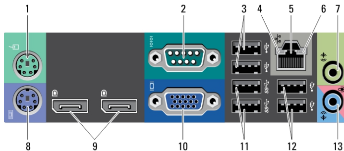
그림 4. 소형 폼팩터의 후면 패널 모습
