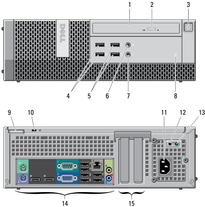
그림 3. 소형 폼팩터의 전면 및 후면 패널 모습
